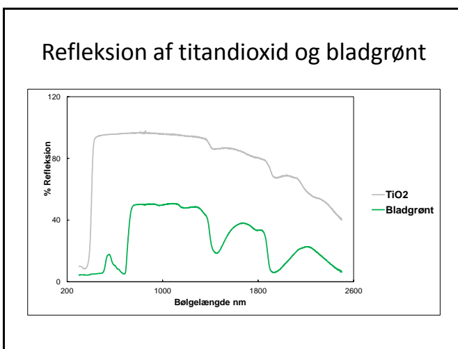
Fig. 8) Titandioxid reflekterer godt både i det synlige område og i NIR. Bladgrønt reflekterer naturligvis grønt lys, men er også ganske effektivt i NIR-området 1
